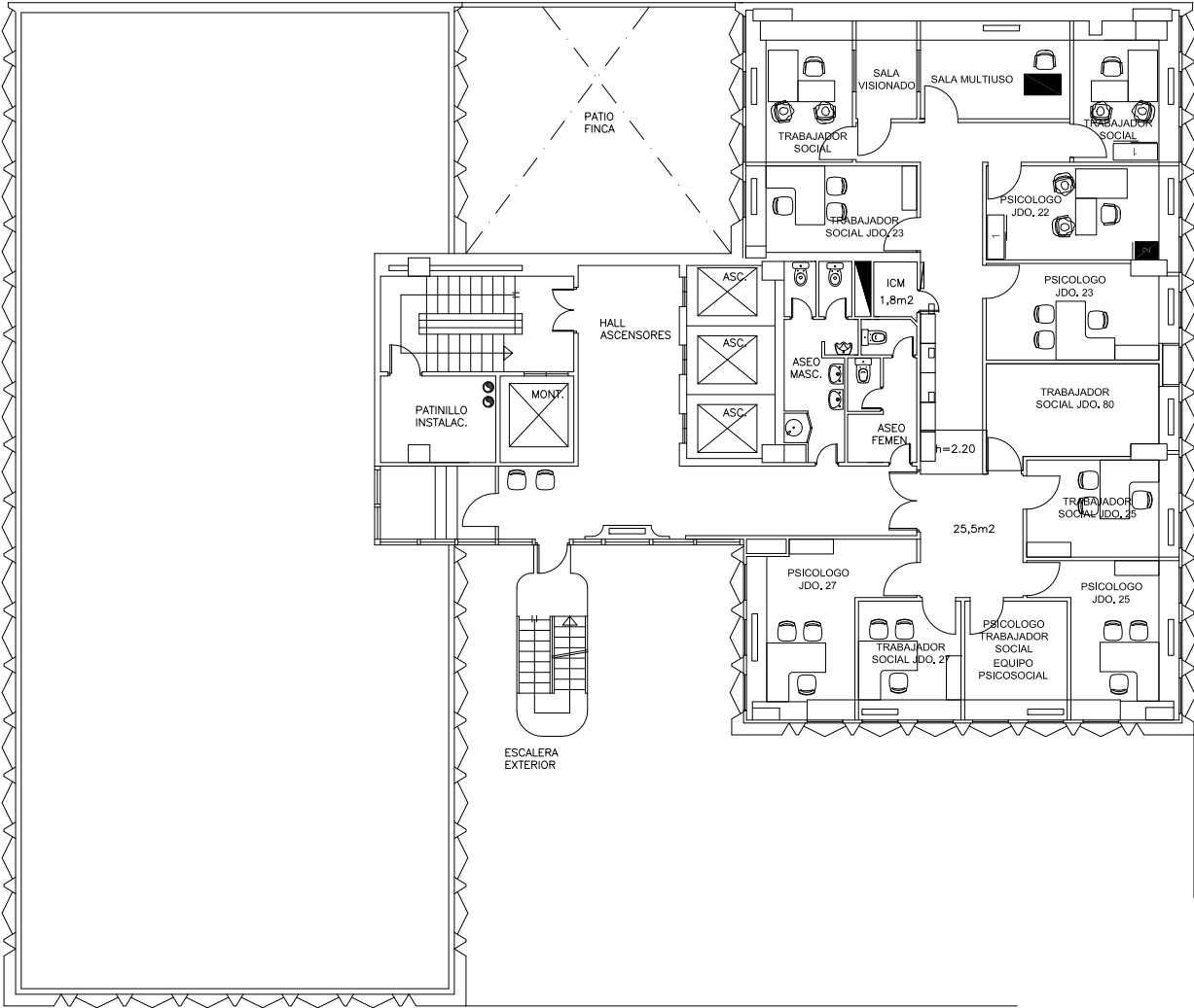
PLANTA DECIMA
